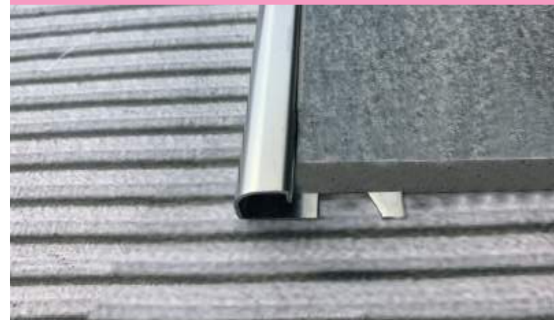
Chiusura perimetrale a pavimento/ Ground covering edging
