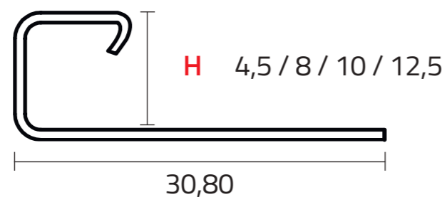
Protezione spigolo / Corner protection
