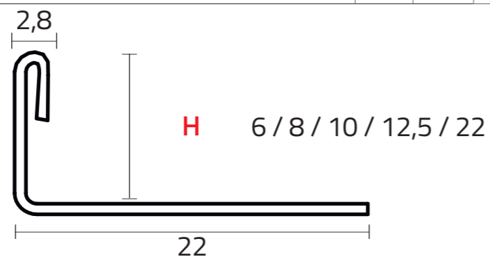
Protezione spigolo/ Corner protection
