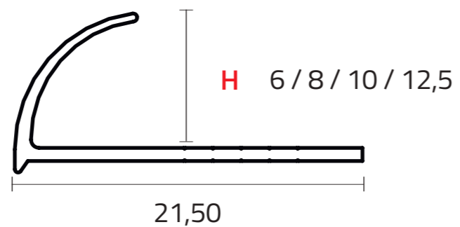
Protezione spigolo/ Corner protection
