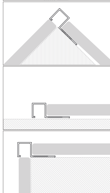
Listello decorativo/ Decorative listello
