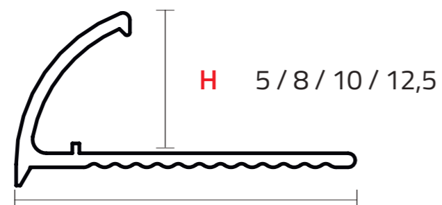
Protezione spigolo/ Corner protection
