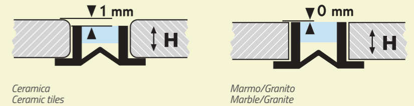
Metodo di posa/Installation method
