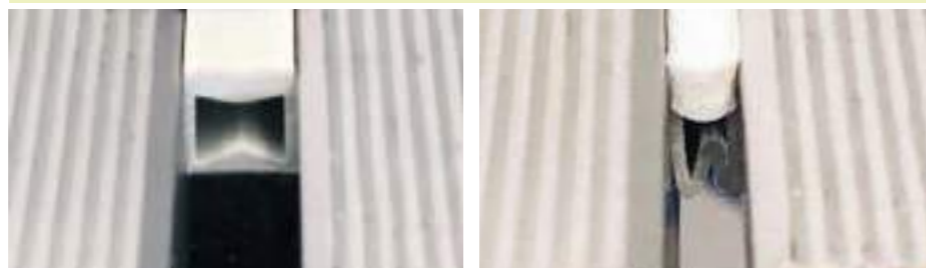
Giunto sottoposto a compressione/ Expansion joint in contraction
