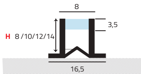
Giunto sottoposto a compressione/ Expansion joint in contraction
